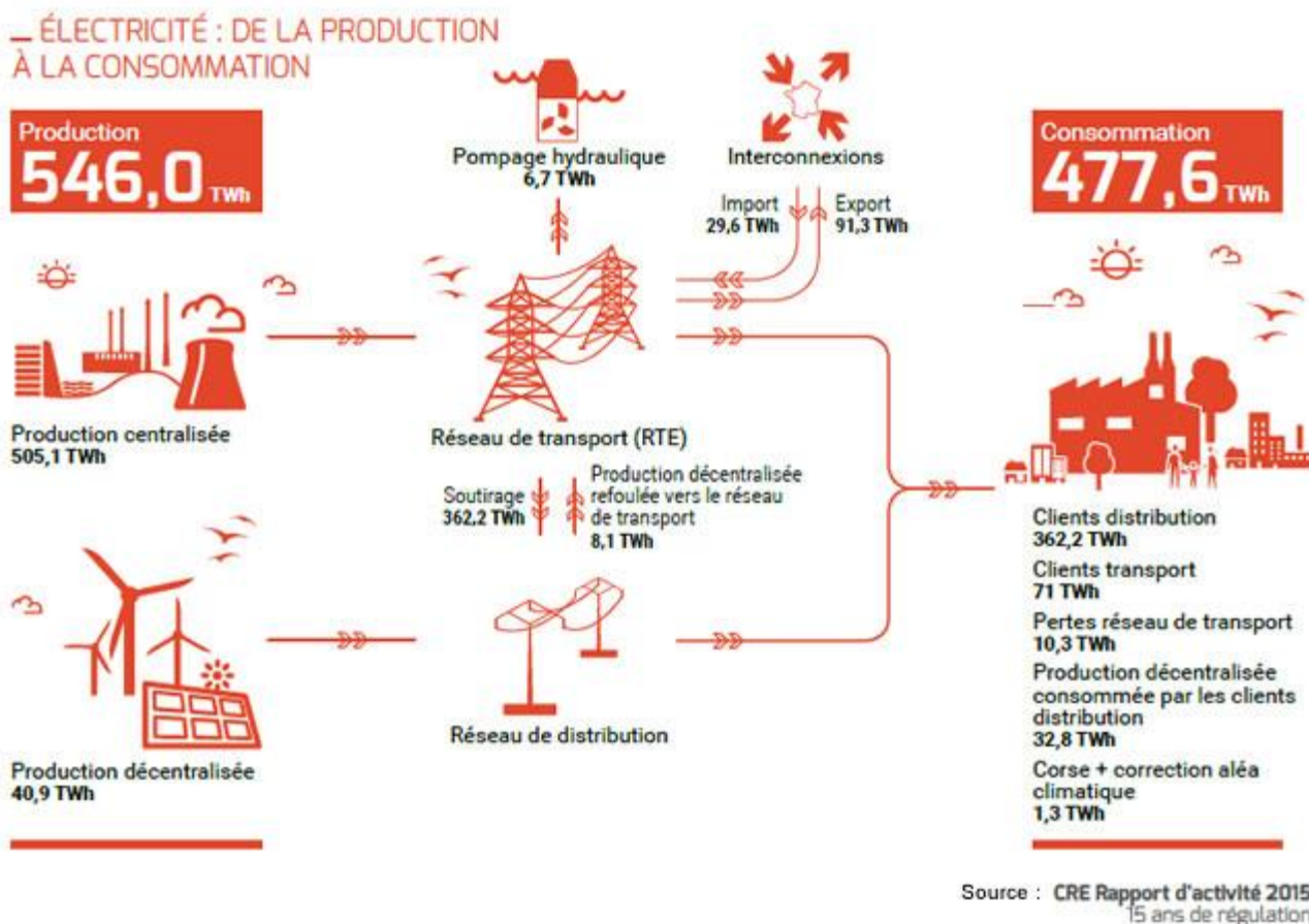
Figure 2 Schéma du système électrique français (source : CRE)
